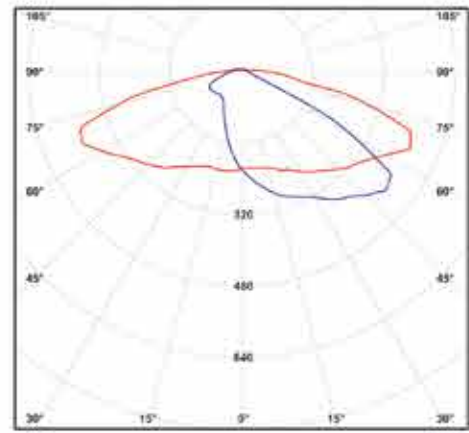
cd/km η=100% — C0 - C180 — C90 - C270
