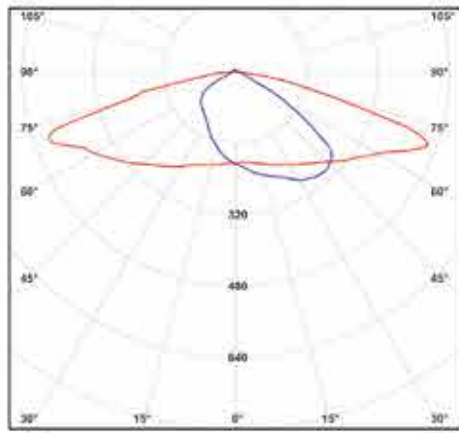
cd/km η=100% — C0 - C180 — C90 - C270
